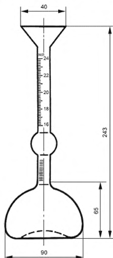
Рисунок 8 — Прибор Ле Шателье
