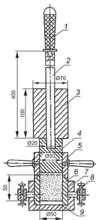
1 — рукоятка; 2 — направляющий стержень; 3 — гиря; 4 — плунжер; 5 — направляющий насадный цилиндр. 6 — разъемный цилиндр; 7 — подставка; 8 — закрепляющие винты; 9 — металлическая пластинка
