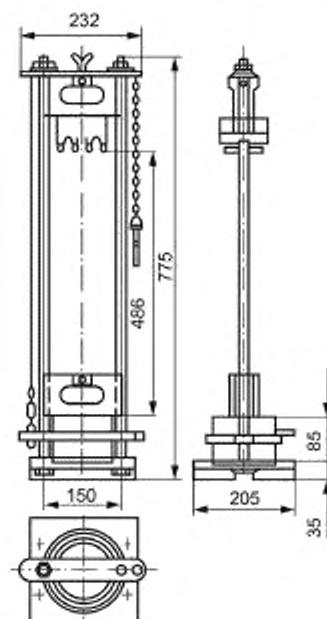
Рисунок 7 — Копер ПМ
