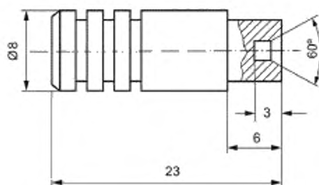
Рисунок 13 — Репер для испытаний
