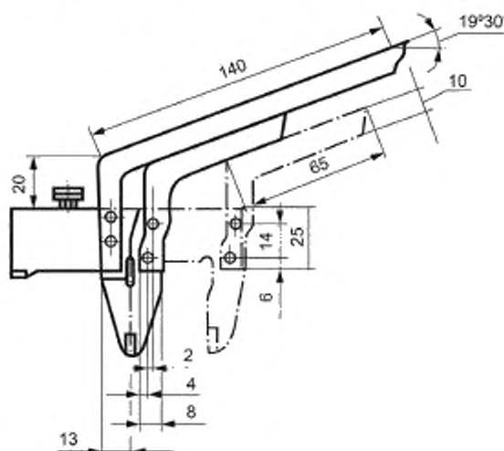
Рисунок 3 — Передвижной шаблон
