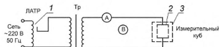
1 — лабораторный регулировочный трансформатор (ЛАТР). 2 — электрод 3 — измерительный куб
